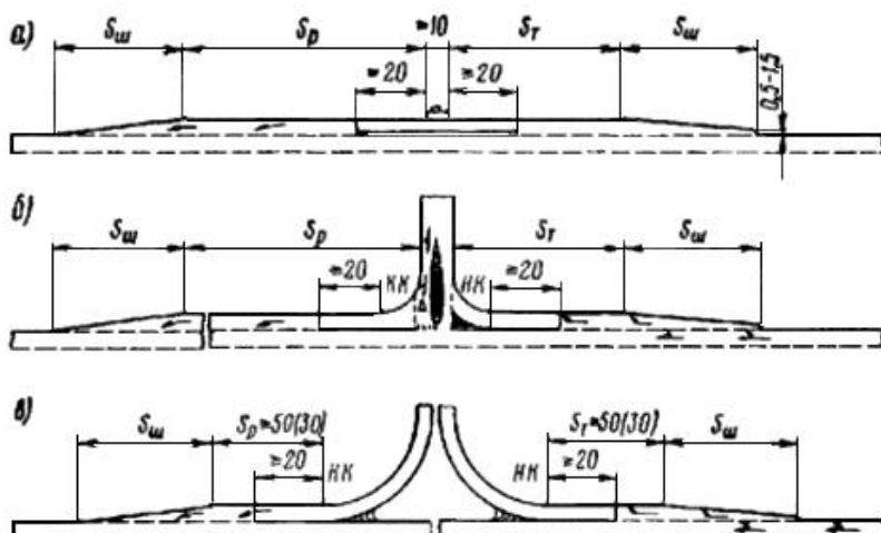
Рисунок 6.7 - Схемы переходно-скоростных полос
